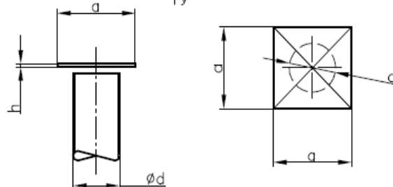
Оголовок монтажный обычный увеличенный "1У"
